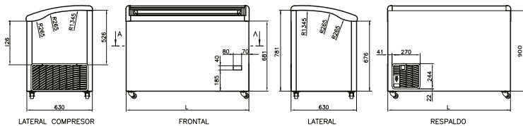
LATERAL COMPRESOR
